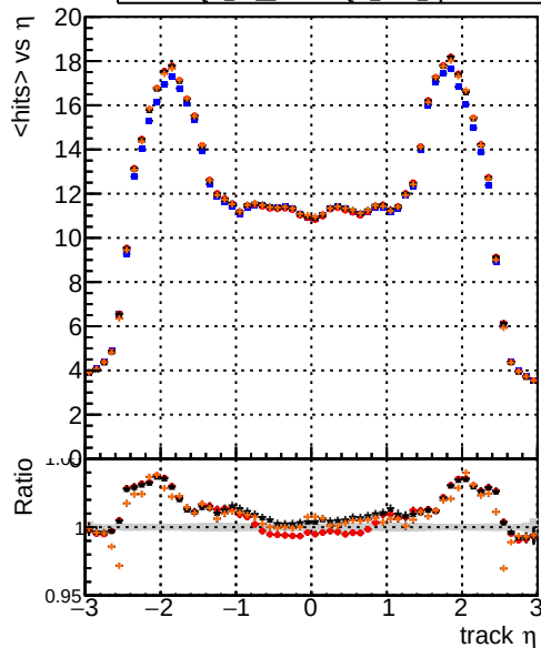
Legend for mean hits vs \eta : Blue line: DQM TT mkFit-DQM original-0 Red line: DQM TT mkFit-DQM original-127 Black line: DQM TT mkFit-DQM mod-127 Orange line: DQM TT mkFit-DQM mod updated-127
