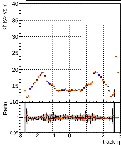
DQM TT mkFit-DQM original-0 DQM TT mkFit-DQM original-127 DQM TT mkFit-DQM mod-127 DQM TT mkFit-DQM mod_updated-127
