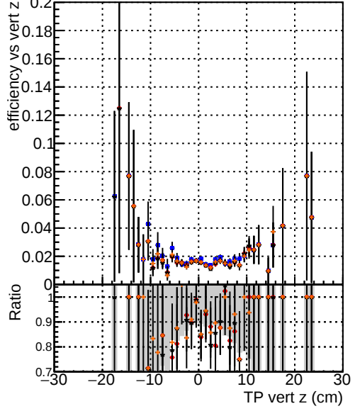
Efficiency vs vert z —●— DQM TT mkFit-DQM original-0 —◆— DQM TT mkFit-DQM original-127 —▲— DQM TT mkFit-DQM mod-127 —×— DQM TT mkFit-DQM mod updated-127
