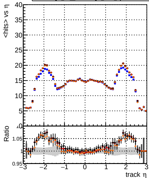
Legend: DQM TT mkFit-DQM original-0 DQM TT mkFit-DQM original-127 DQM TT mkFit-DQM mod-127 DQM TT mkFit-DQM mod updated-127
