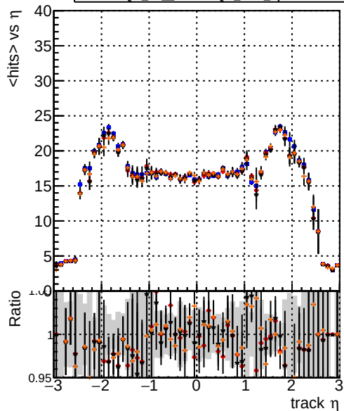
mean hits DQM TT mkFit-DQM original-0 DQM TT mkFit-DQM original-127 DQM TT mkFit-DQM mod-127 DQM TT mkFit-DQM mod updated-127
