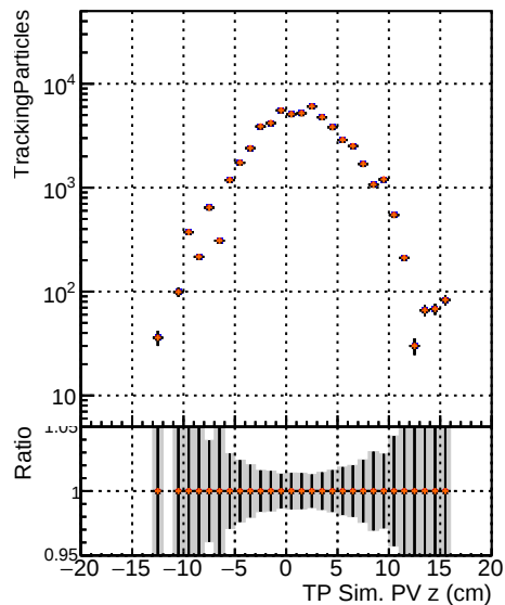
N of simulated tracks vs. sim PV z 1000 2000 3000 4000 5000 6000 7000 8000 9000 10000 11000 12000 13000 14000 15000 16000 17000 18000 19000 20000 21000 22000 23000 24000 25000 26000 27000 28000 29000 30000 31000 32000 33000 34000 35000 36000 37000 38000 39000 40000 41000 42000 43000 44000 45000 46000 47000 48000 49000 50000 51000 52000 53000 54000 55000 56000 57000 58000 59000 60000 61000 62000 63000 64000 65000 66000 67000 68000 69000 70000 71000 72000 73000 74000 75000 76000 77000 78000 79000 80000 81000 82000 83000 84000 85000 86000 87000 88000 89000 90000 91000 92000 93000 94000 95000 96000 97000 98000 99000 100000
