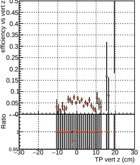
Efficiency vs vertpos —●— DQM TT mkFit-DQM_original-0 —●— DQM TT mkFit-DQM_original-127 —●— DQM TT mkFit-DQM_mod-127 —●— DQM TT mkFit-DQM_mod_updated-127
