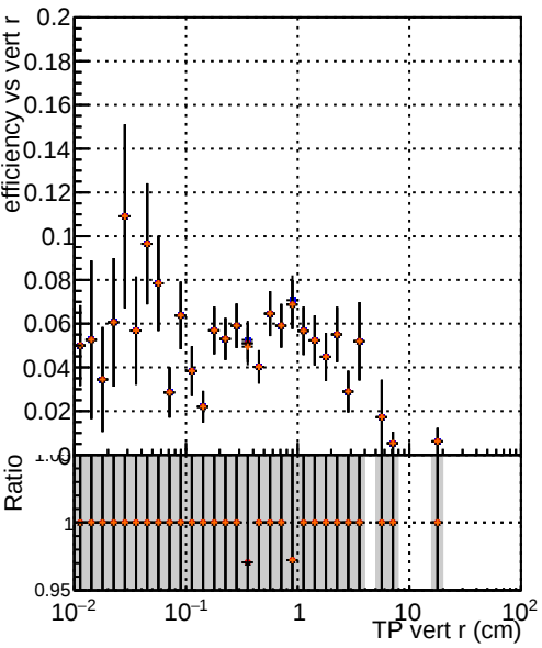
Efficiency vs vertpos —●— DQM TT mkFit-DQM_original-0 —●— DQM TT mkFit-DQM_original-127 —●— DQM TT mkFit-DQM_mod-127 —●— DQM TT mkFit-DQM_mod_updated-127
