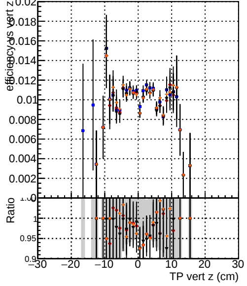
Efficiency vs. sim PV z —●— DQM TT mkFit-DQM original-0 —▲— DQM TT mkFit-DQM original-127 —▼— DQM TT mkFit-DQM mod-127 —◆— DQM TT mkFit-DQM mod_updated-127
