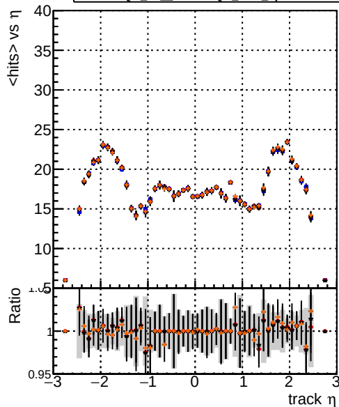
mean hit DQM TT mkFit-DQM original-0 DQM TT mkFit-DQM original-127 DQM TT mkFit-DQM mod-127 DQM TT mkFit-DQM mod updated-127
