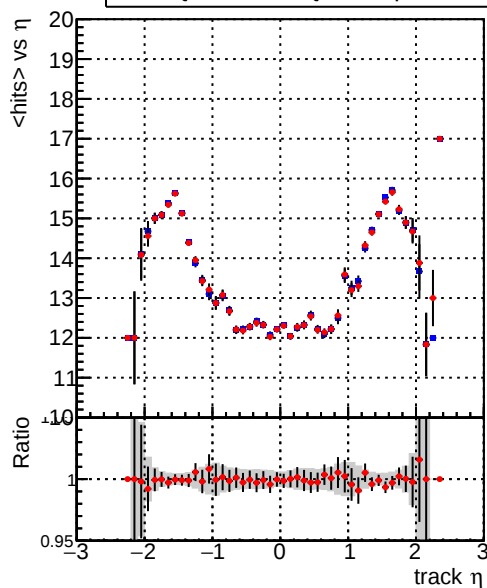
— DQM_TT_mkFit-DQM_mod-127 — DQM_TT_mkFit-DQM_mod_updated-127
