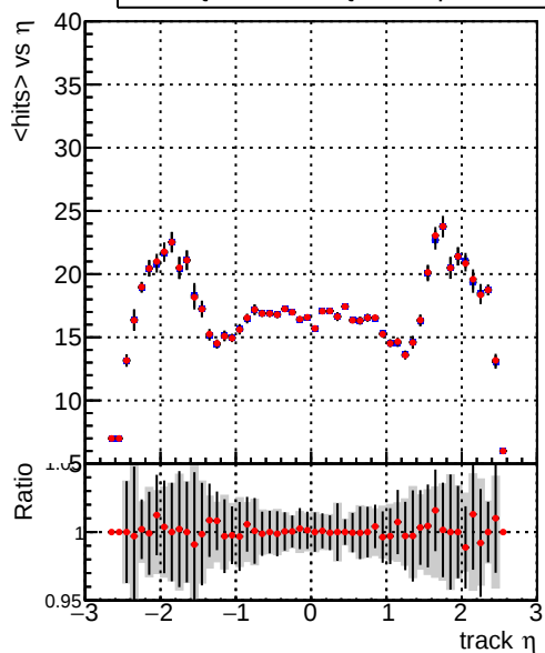
— DQM_TT_mkFit-DQM_mod-127 — DQM_TT_mkFit-DQM_mod_updated-127
