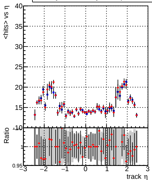
— DQM_TT_mkFit-DQM_mod-127 — DQM_TT_mkFit-DQM_mod_updated-127
