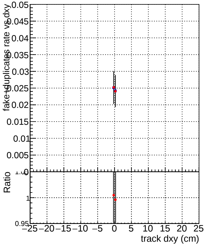
DQM_TT__mkFit-DQM_mod-127 DQM_TT__mkFit-DQM_mod_updated-127
