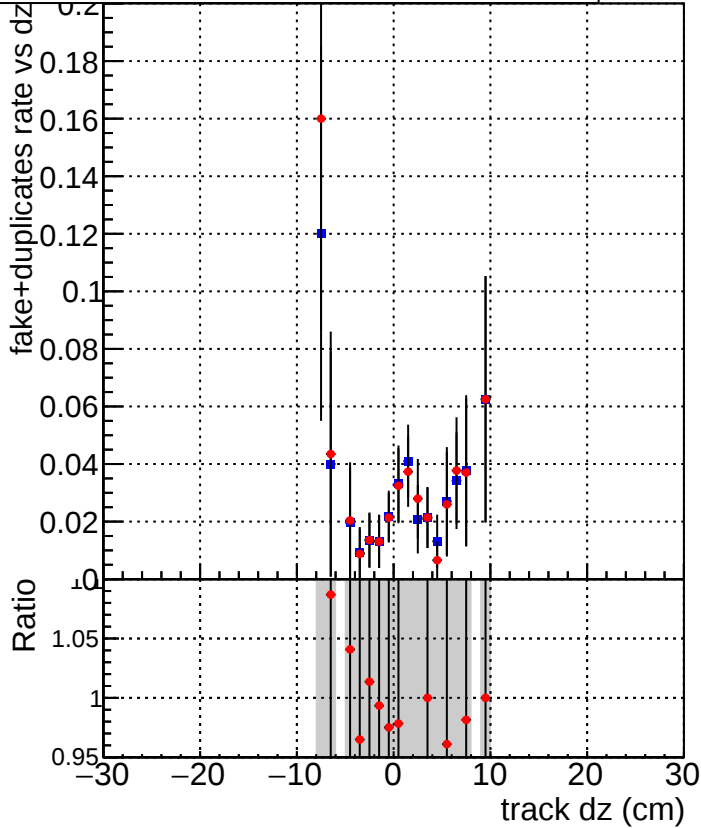
DQM_TT__mkFit-DQM_mod-127 DQM_TT__mkFit-DQM_mod_updated-127
