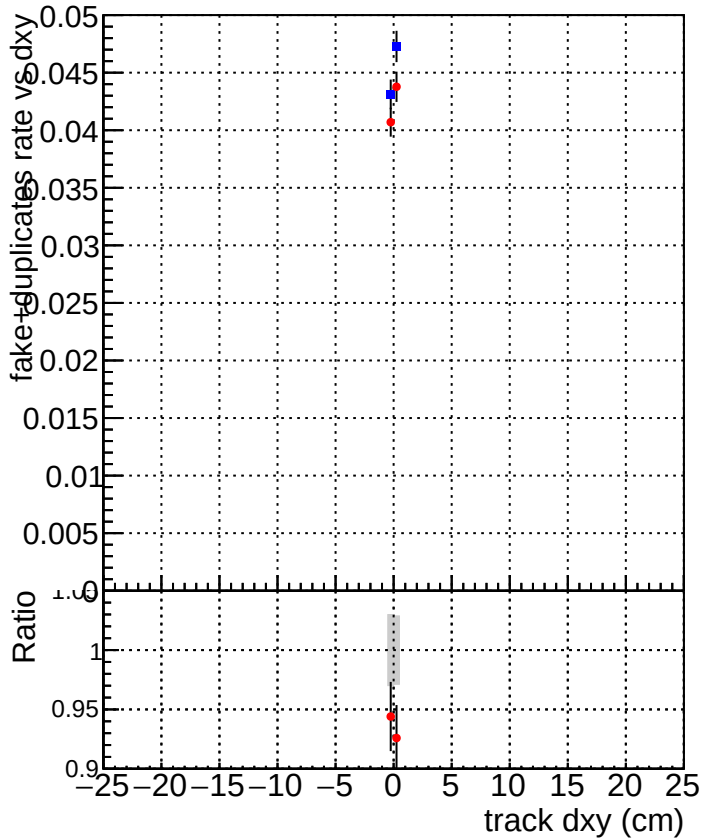
DQM_TT_mkFit-DQM_mod-127 DQM_TT_mkFit-DQM_mod_updated-127
