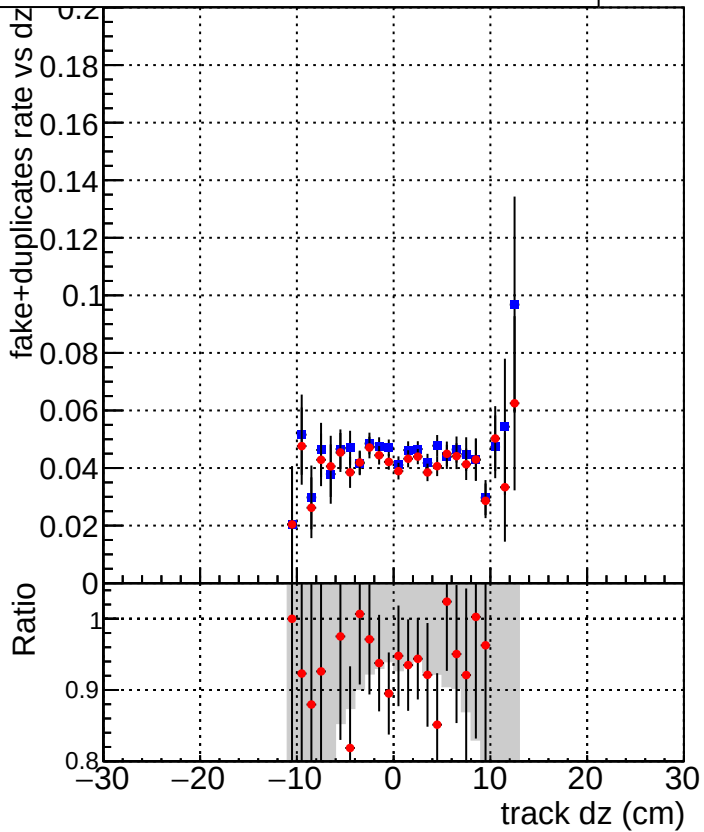
DQM_TT_mkFit-DQM_mod-127 DQM_TT_mkFit-DQM_mod_updated-127
