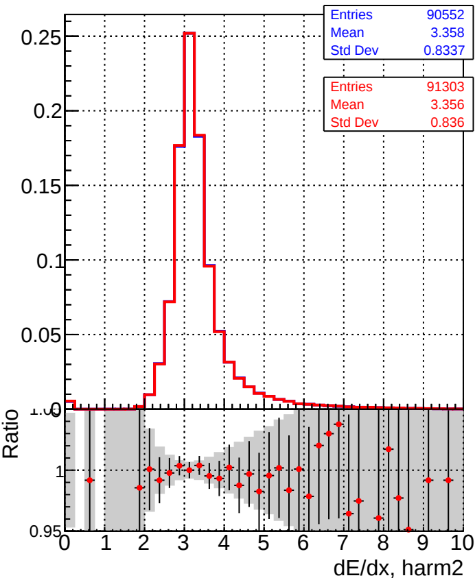
DQM_TT_mkFit-DQM_mod-127 DQM_TT_mkFit-DQM_mod_updated-127
