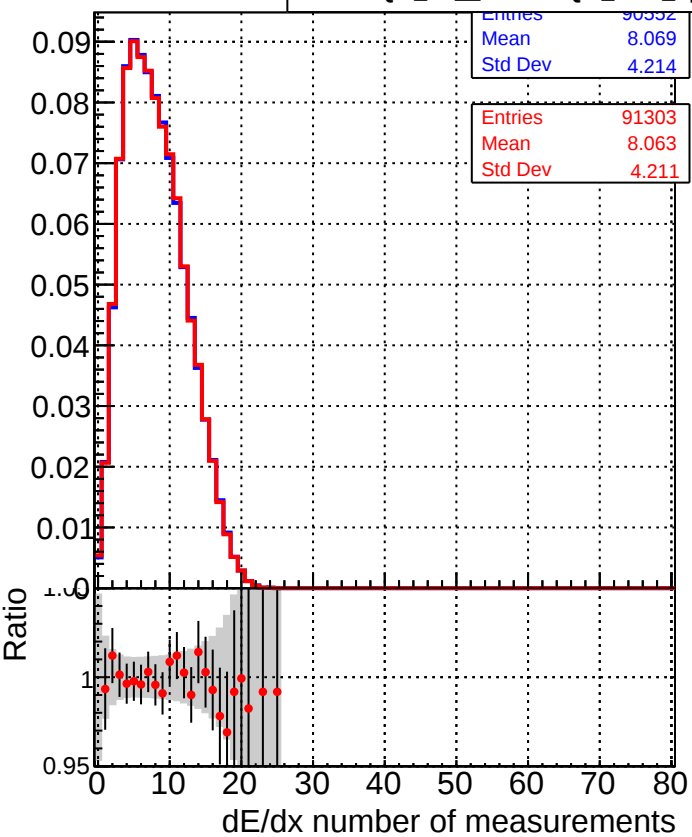
DQM_TT_mkFit-DQM_mod-127 DQM_TT_mkFit-DQM_mod_updated-127
