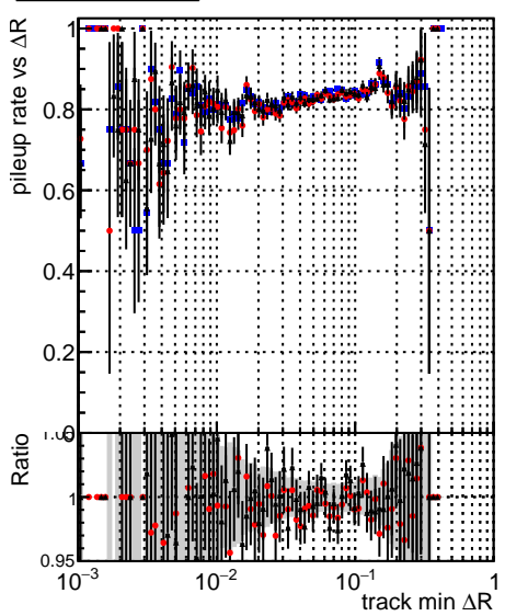
Legend for all plots: —●— DQM TT mkFit-DQM original-0 —●— DQM TT mkFit-DQM mod-127 —●— DQM TT mkFit-DQM mod_updated-127
