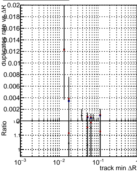
Legend for all plots: —●— DQM TT mkFit-DQM original-0 —●— DQM TT mkFit-DQM mod-127 —●— DQM TT mkFit-DQM mod_updated-127
