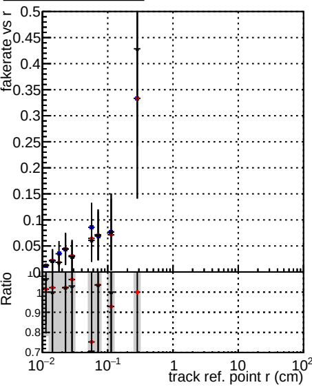
Fake rate vs verpos DQM TT mkFit-DQM original-0 DQM TT mkFit-DQM mod-127 DQM TT mkFit-DQM mod-updated-127
