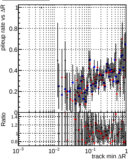
Legend: DQM TT mkFit-DQM original-0 (blue dots), DQM TT mkFit-DQM mod-127 (red dots), DQM TT mkFit-DQM mod-updated-127 (black dots), DQM TT mkFit-DQM mod-updated-127 (grey dots)
