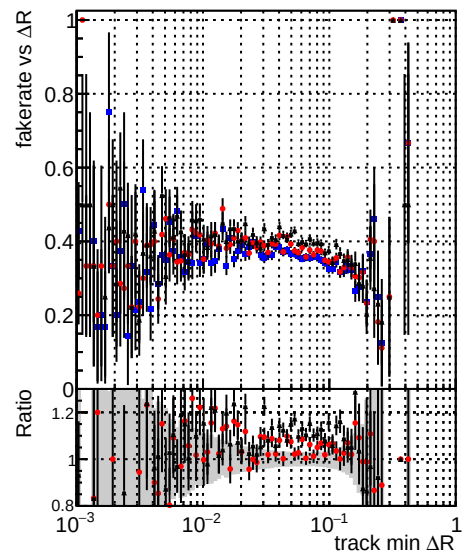
—●— DQM TT mkFit-DQM original-0 —●— DQM TT mkFit-DQM mod-127 —●— DQM TT mkFit-DQM mod-127
