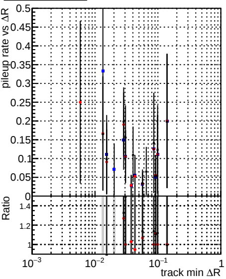
Legend: DQM TT mkFit-DQM original-0 (black), DQM TT mkFit-DQM mod-127 (red), DQM TT mkFit-DQM mod-updated-127 (grey)
