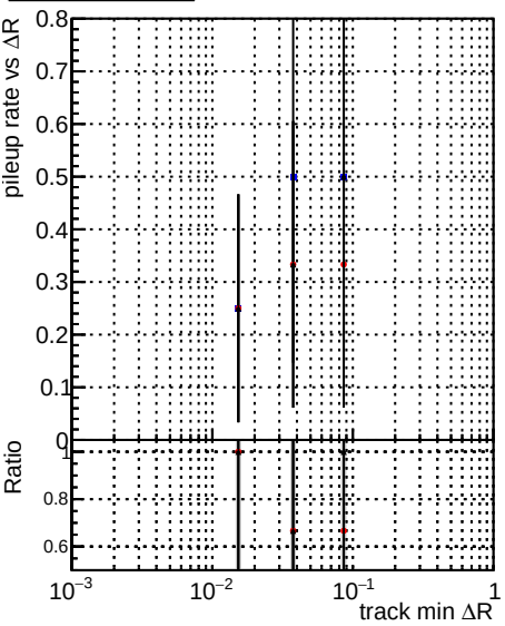
Legend: DQM TT mkFit-DQM original-0 (blue), DQM TT mkFit-DQM original-127 (red), DQM TT mkFit-DQM updated-127 (black)
