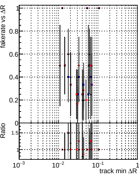
Legend: DQM TT mkFit-DQM original-0 (blue), DQM TT mkFit-DQM original-127 (red), DQM TT mkFit-DQM updated-127 (black)
