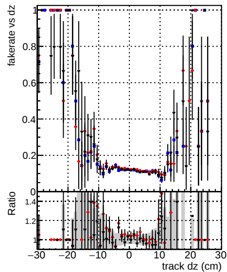
DOM TT mkFit-DOM-original-0 DOM TT mkFit-DOM-updated-127
