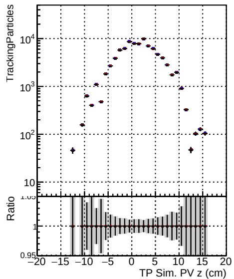
N of simulated tracks vs. sim PV z 0 1 1 1 2 1 3 1 4 1 5 1 6 1 7 1 8 1 9 1 10 1 11 1 12 1 13 1 14 1 15 1 16 1 17 1 18 1 19 1 20 1 21 1 22 1 23 1 24 1 25 1 26 1 27 1 28 1 29 1 30 1 31 1 32 1 33 1 34 1 35 1 36 1 37 1 38 1 39 1 40 1 41 1 42 1 43 1 44 1 45 1 46 1 47 1 48 1 49 1 50 1 51 1 52 1 53 1 54 1 55 1 56 1 57 1 58 1 59 1 60 1 61 1 62 1 63 1 64 1 65 1 66 1 67 1 68 1 69 1 70 1 71 1 72 1 73 1 74 1 75 1 76 1 77 1 78 1 79 1 80 1 81 1 82 1 83 1 84 1 85 1 86 1 87 1 88 1 89 1 90 1 91 1 92 1 93 1 94 1 95 1 96 1 97 1 98 1 99 1 100 1 101 1 102 1 103 1 104 1 105 1 106 1 107 1 108 1 109 1 110 1 111 1 112 1 113 1 114 1 115 1 116 1 117 1 118 1 119 1 120 1 121 1 122 1 123 1 124 1 125 1 126 1 127 1 128 1 129 1 130 1 131 1 132 1 133 1 134 1 135 1 136 1 137 1 138 1 139 1 140 1 141 1 142 1 143 1 144 1 145 1 146 1 147 1 148 1 149 1 150 1 151 1 152 1 153 1 154 1 155 1 156 1 157 1 158 1 159 1 160 1 161 1 162 1 163 1 164 1 165 1 166 1 167 1 168 1 169 1 170 1 171 1 172 1 173 1 174 1 175 1 176 1 177 1 178 1 179 1 180 1
