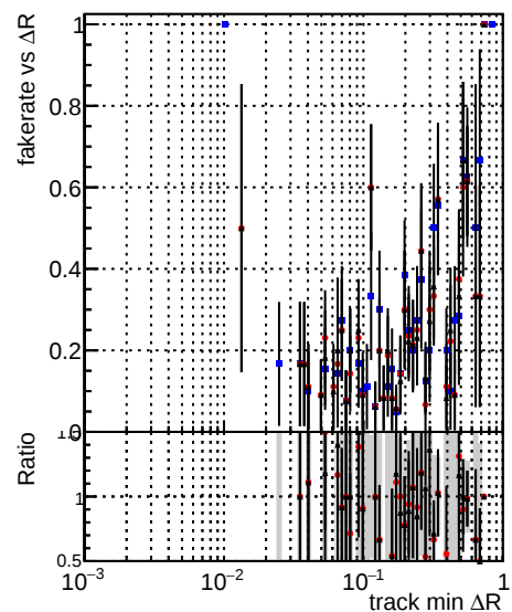
—●— DQM TT mkFit-DQM original-0 —●— DQM TT mkFit-DQM original-127 —●— DQM TT mkFit-DQM mod-127
