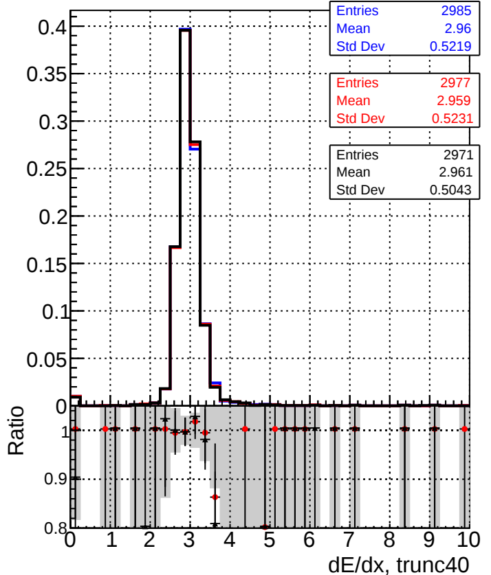
dE/dx estimator 2
