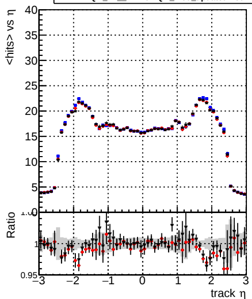
— DQM_TT_mkFit-DQM_original-0 — DQM_TT_mkFit-DQM_mod-127 — DQM_TT_mkFit-DQM_mod_updatedmod-127
