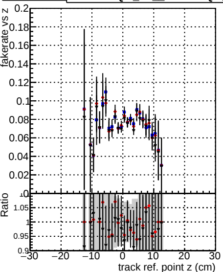
— — — — — — — — Fake rate vs v DQM TT mkFit-DQM original-0 DQM TT mkFit-DQM mod-127 DQM TT mkFit-DQM mod-updatedmod-127
