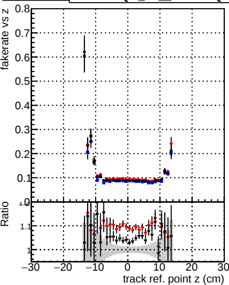
Fake rate vs verpos Legend: DQM TT mkFit-DQM original-0 (blue circles) DQM TT mkFit-DQM mod-127 (red circles) DQM TT mkFit-DQM mod_updatedmod-127 (black circles)
