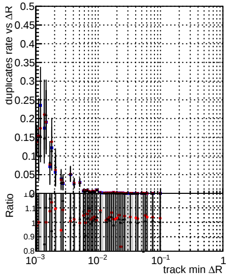
—●— DQM TT mkFit-DQM original-0 —●— DQM TT mkFit-DQM mod-127 —●— DQM TT mkFit-DQM mod-updatedmod-127
