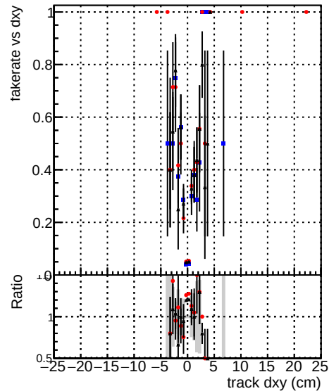
DOM TT mkFit-DOM-original-0 DOM TT mkFit-DOM-mod-127 DOM TT mkFit-DOM-mod-updatedmod-127
