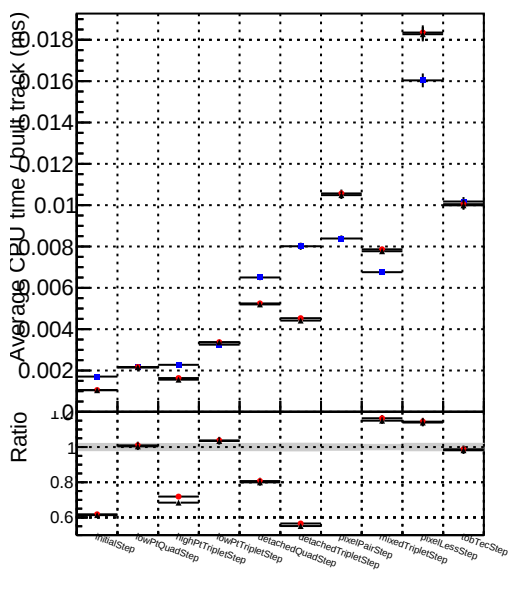
Average CPU time / built track 1 0.000000 2 0.000000 3 0.000000 4 0.000000 5 0.000000 6 0.000000 7 0.000000 8 0.000000 9 0.000000 10 0.000000 11 0.000000 12 0.000000 13 0.000000 14 0.000000 15 0.000000 16 0.000000 17 0.000000 18 0.000000 19 0.000000 20 0.000000 21 0.000000 22 0.000000 23 0.000000 24 0.000000 25 0.000000 26 0.000000 27 0.000000 28 0.000000 29 0.000000 30 0.000000 31 0.000000 32 0.000000 33 0.000000 34 0.000000 35 0.000000 36 0.000000 37 0.000000 38 0.000000 39 0.000000 40 0.000000 41 0.000000 42 0.000000 43 0.000000 44 0.000000 45 0.000000 46 0.000000 47 0.000000 48 0.000000 49 0.000000 50 0.000000 51 0.000000 52 0.000000 53 0.000000 54 0.000000 55 0.000000 56 0.000000 57 0.000000 58 0.000000 59 0.000000 60 0.000000 61 0.000000 62 0.000000 63 0.000000 64 0.000000 65 0.000000 66 0.000000 67 0.000000 68 0.000000 69 0.000000 70 0.000000 71 0.000000 72 0.000000 73 0.000000 74 0.000000 75 0.000000 76 0.000000 77 0.000000 78 0.000000 79 0.000000 80 0.000000 81 0.000000 82 0.000000 83 0.000000 84 0.000000 85 0.000000 86 0.000000 87 0.000000 88 0.000000 89 0.000000 90 0.000000 91 0.000000 92 0.000000 93 0.000000 94 0.000000 95 0.000000 96 0.000000 97 0.000000 98 0.000000 99 0.000000 100 0.000000
