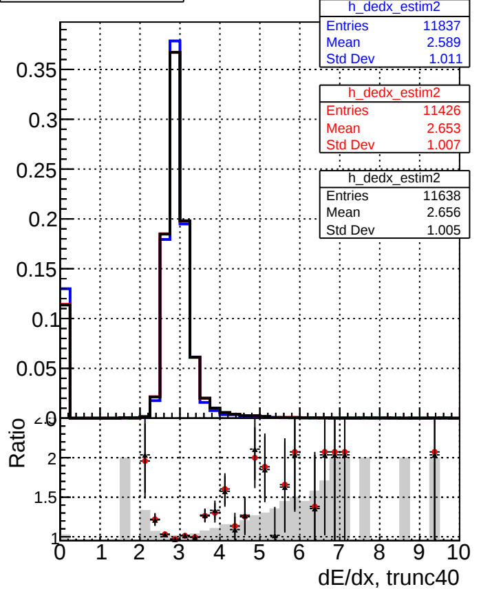
dE/dx estimator 2
