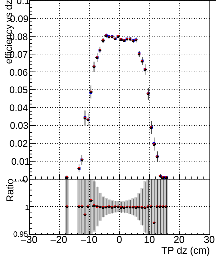
Efficiency vs Dz ■ DQM_mkFit_newBASE3 ● DQM_mkFit_new ▲ DQM_mkFit_newANDPL
