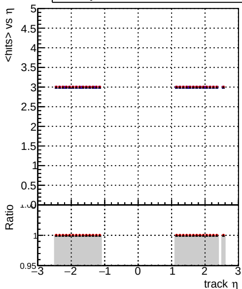
mean hits — DQM_mkFit_newBASE3 — DQM_mkFit_new — DQM_mkFit_newANDPL
