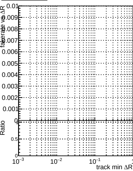
Fake rate vs \Delta R(\text{track, jet}) Legend: DQM_mkFit_newBASE3 DQM_mkFit_new DQM_mkFit_newANDPL
