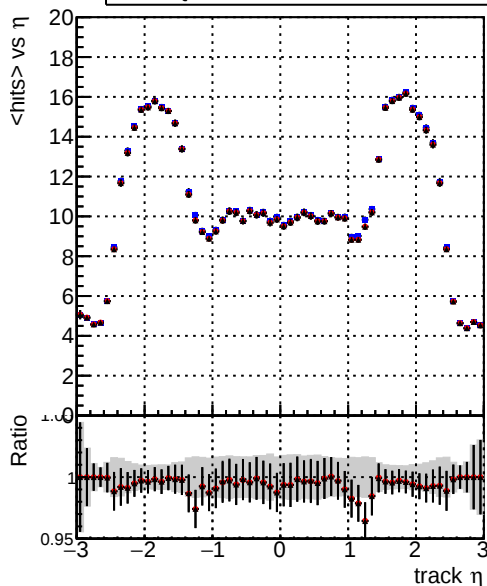
mean hits — DQM_mkFit_newBASE3 — DQM_mkFit_new — DQM_mkFit_newANDPL
