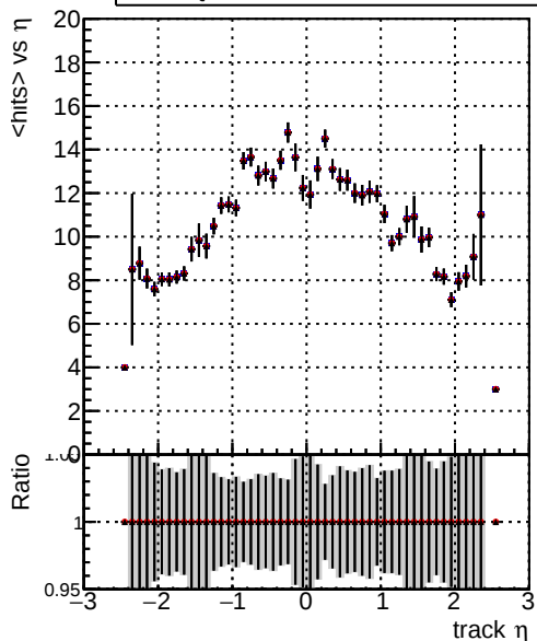
mean hit — DQM_mkFit_newBASE3 — DQM_mkFit_new — DQM_mkFit_newANDPL
