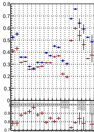
Fake rate vs. —●— DQM TT mkFit BDT —●— DQM TT mkFit
