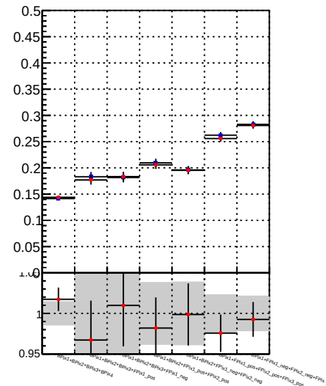
Fake rate vs. DQM TT mkFit BDT DQM TT mkFit
