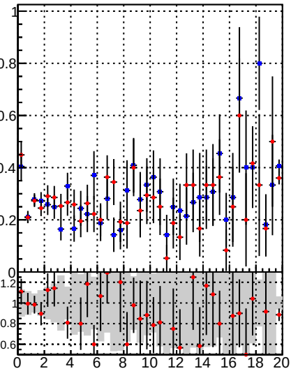
Fake rate vs. DQM TT mkFit BDT DQM TT mkFit
