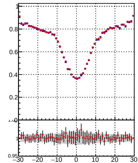
—■— DQM TT mkFit —●— DQM TT mkFit_BDT
