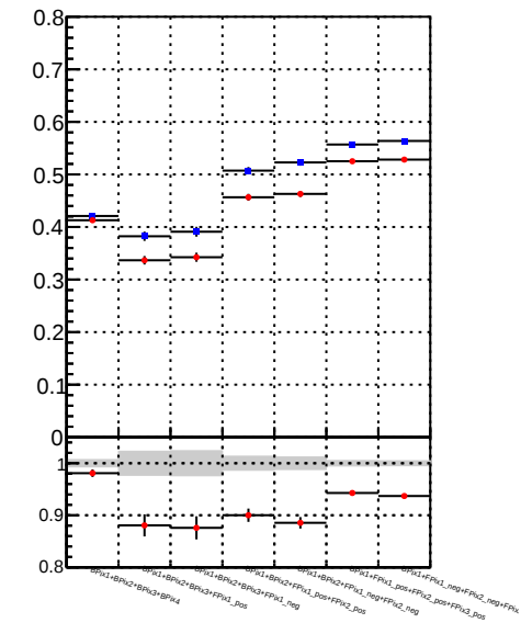
Fake rate vs. DQM TT mkFit DQM TT mkFit BDT
