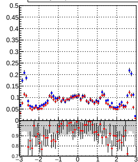
— DQM_DisplacedSUSY_mkFit_BDT_ — DQM_DisplacedSUSY_mkFit_
