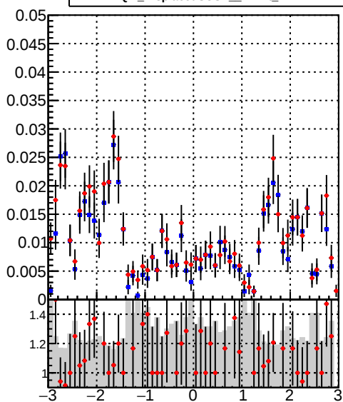
■ DQM_DisplacedSUSY_mkFit_BDT_ ■ DQM_DisplacedSUSY_mkFit_
