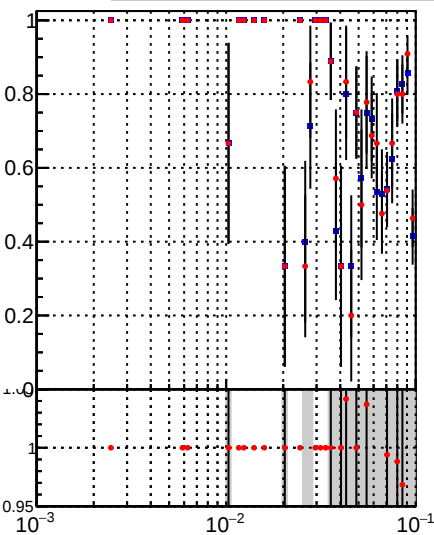
—•— DQM_DisplacedSUSY_mkFit_BDT_ —•— DQM_DisplacedSUSY_mkFit_
