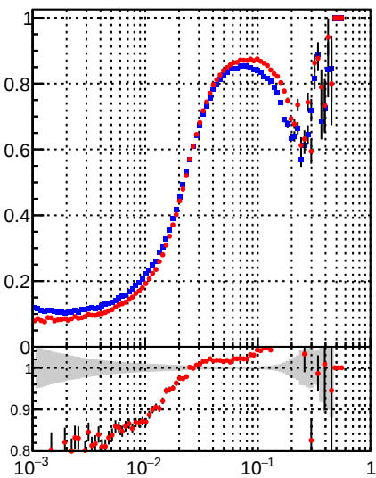
—•— DQM_DisplacedSUSY_mkFit_BDT_ —•— DQM_DisplacedSUSY_mkFit_
