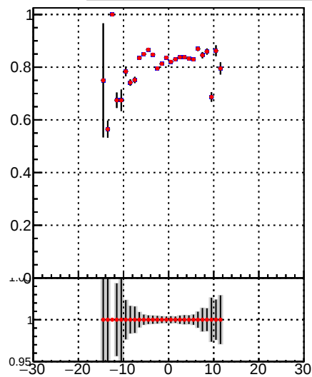
—•— DQM_DisplacedSUSY_mkFit_BDT_ —•— DQM_DisplacedSUSY_mkFit_
