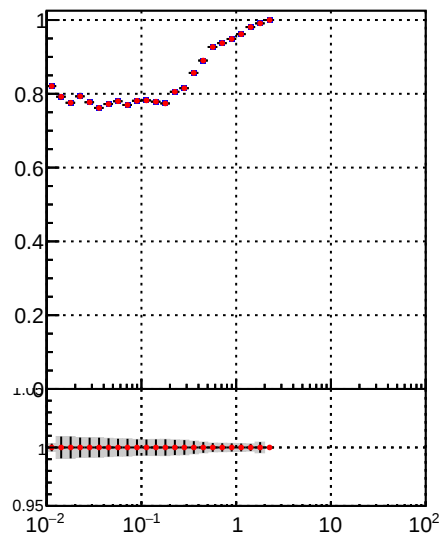
—•— DQM_DisplacedSUSY_mkFit_BDT_ —•— DQM_DisplacedSUSY_mkFit_
