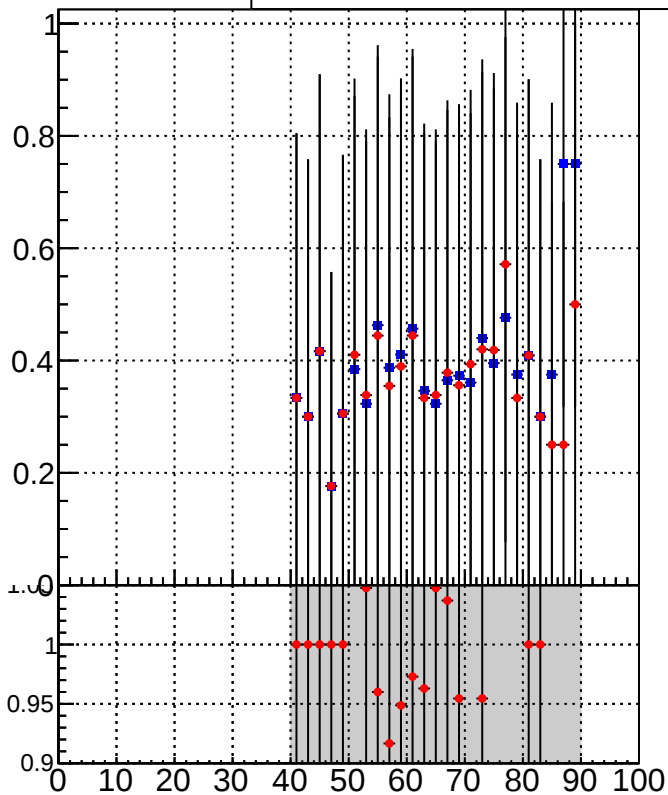
■ DQM_DisplacedSUSY_mkFit_BDT_ ● DQM_DisplacedSUSY_mkFit_
