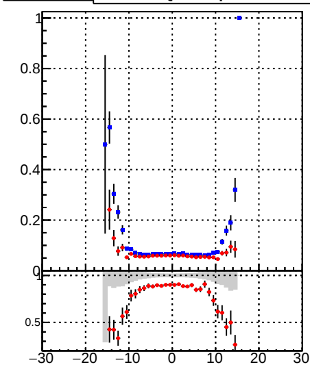
—●— DQM_DisplacedSUSY_mkFit_BDT_ —●— DQM_DisplacedSUSY_mkFit_
