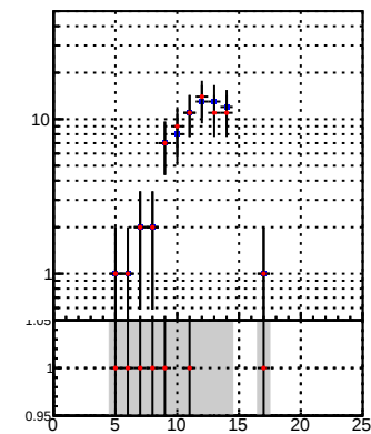
—●— DQM_DisplacedSUSY_mkFit_BDT_ —●— DQM_DisplacedSUSY_mkFit_
