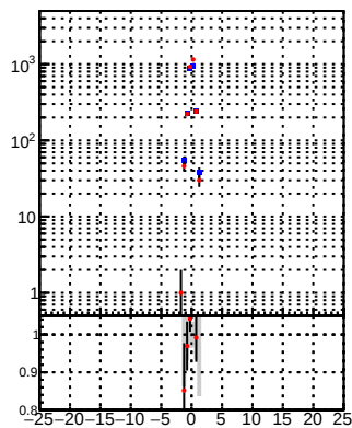
—•— DQM_DisplacedSUSY_mkFit_
