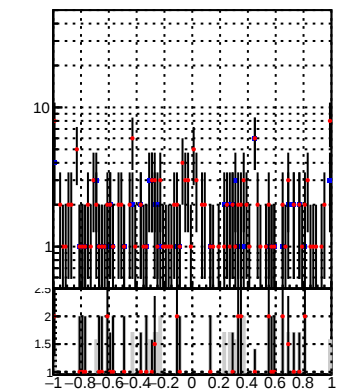
—•— DQM_DisplacedSUSY_mkFit_
