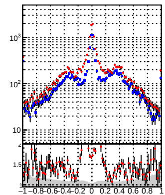
—•— DQM_DisplacedSUSY_mkFit_
